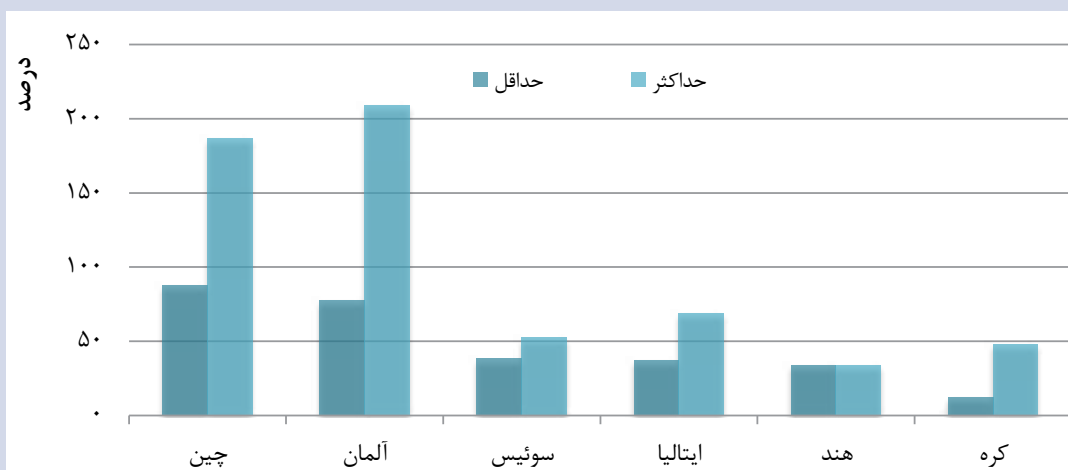
نمودار ۱ - حاشیه دامپینگ در ایالات متحده - ۱۰ می ۲۰۱۷
